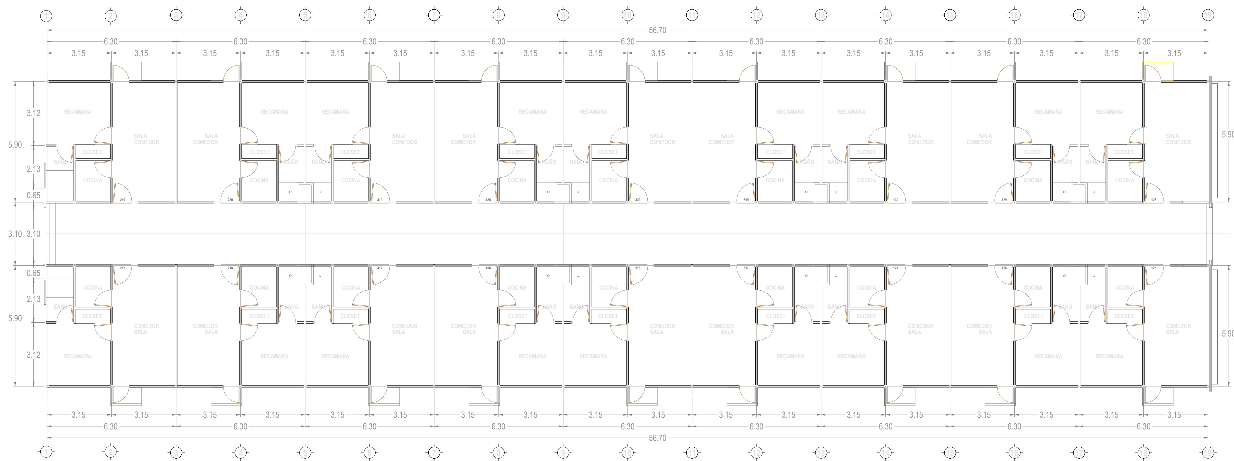
PLANTA 4to PISO
