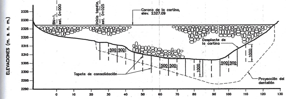
CADENAMIENTO (m) PERFIL LONGITUDINAL POR EL EJE DE LA CORTINA ESC. 1:500
