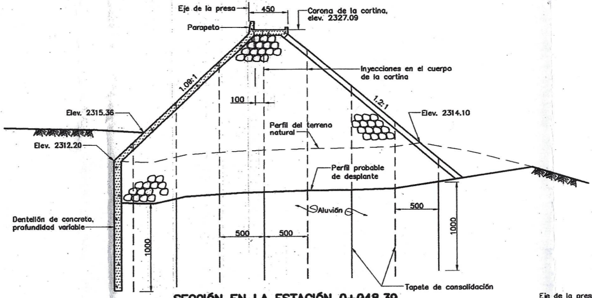
SECCIÓN EN LA ESTACIÓN 0+048.39 SEGUN CORTE A-A ESC. 1:200
