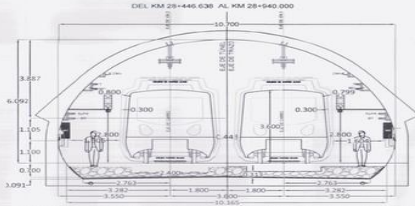
SECCIÓN TIPO S1 DE PROYECTO EN ZONA ACTUALMENTE CONSTRUIDA ACOTACIÓN: m ESCALA: 1:100 Ver Nota 11
