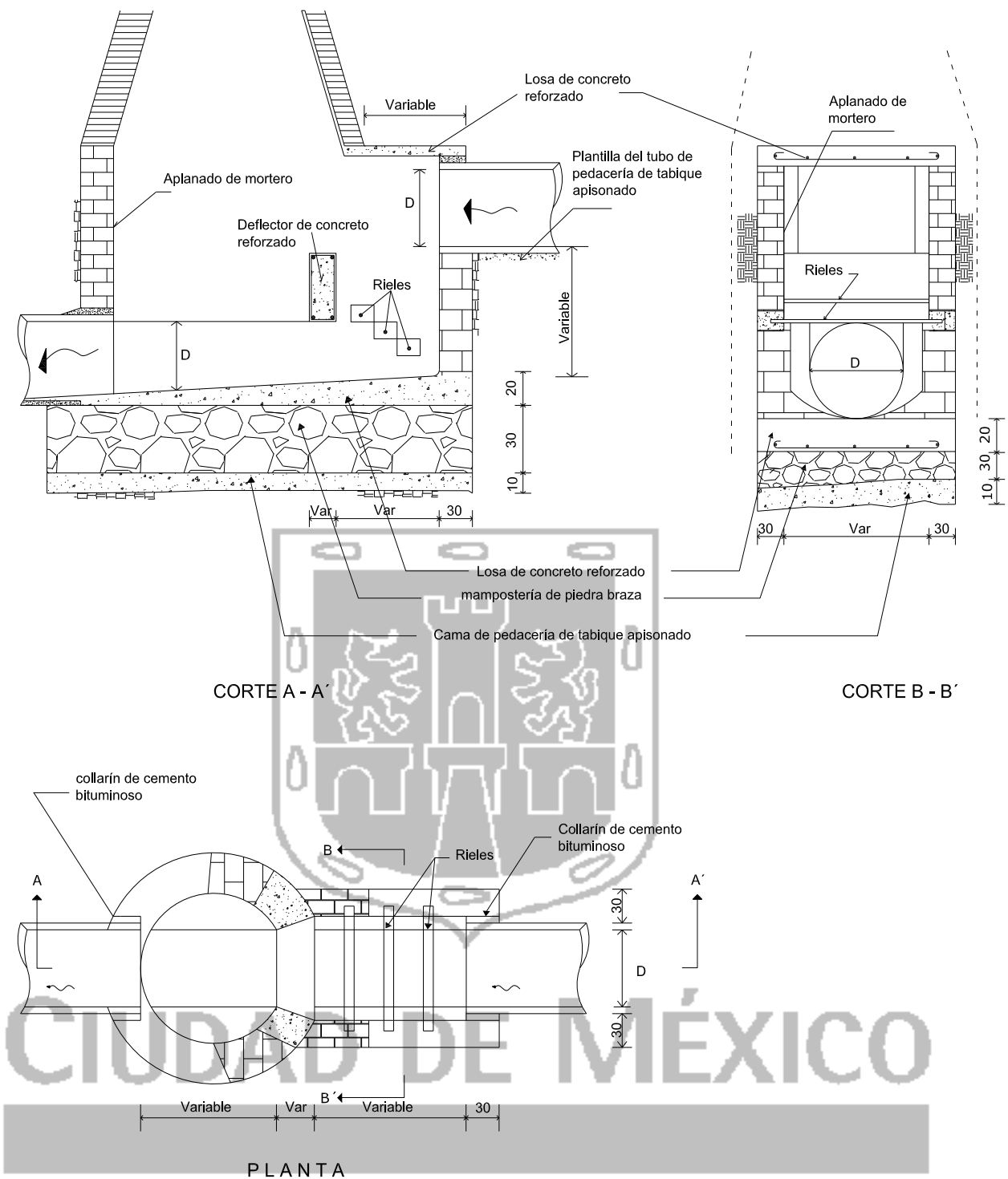
FIGURA 8.- Pozo caja de visita con caída y deflector
