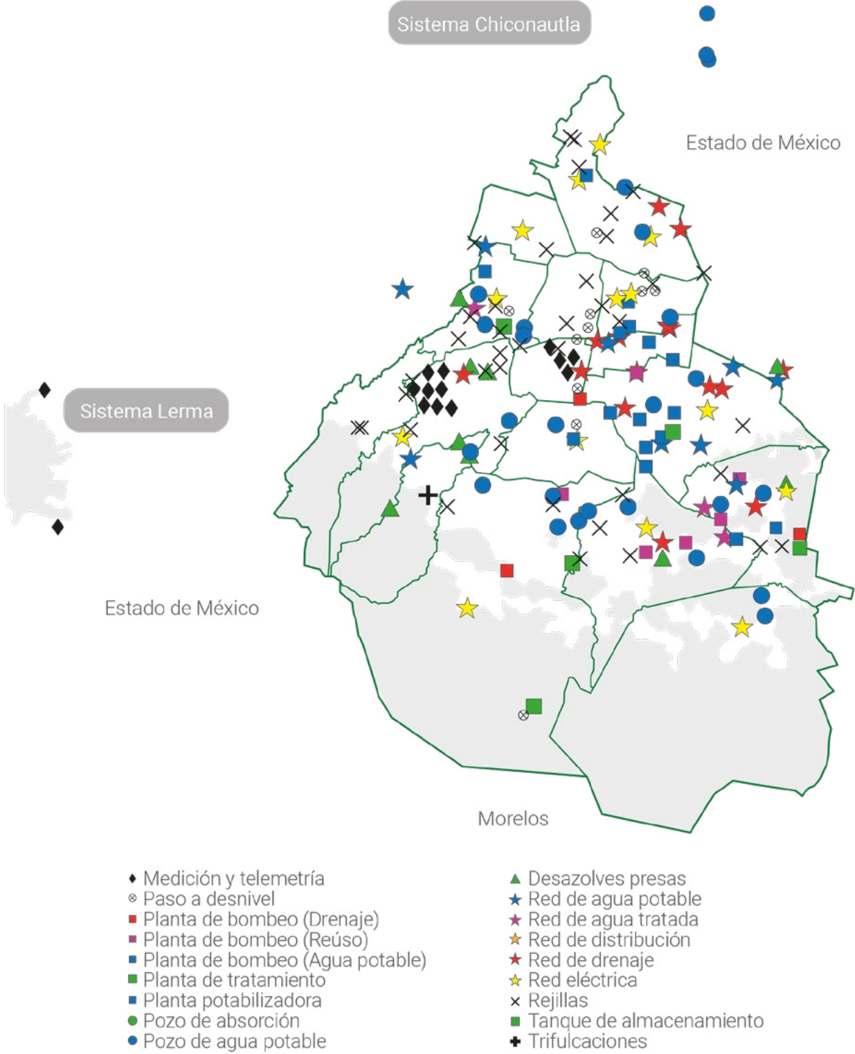
MAPA DE OBRAS HIDRÁULICAS EJECUTADAS POR TIPO DE INFRAESTRUCTURA, 2025
