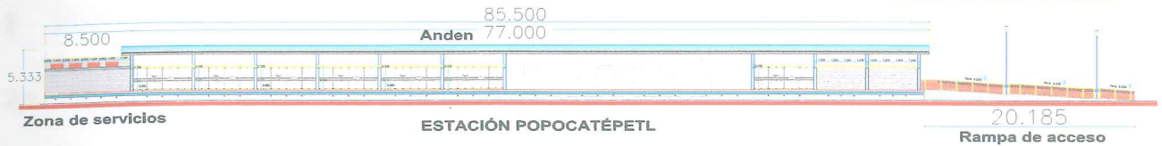
Figura 1.3. Vista en corte de la estación Popocatepetl, tomando como referencia la información de las estaciones Eugenia, División del Norte y Terminal Xoco (CEMEX 2019)
