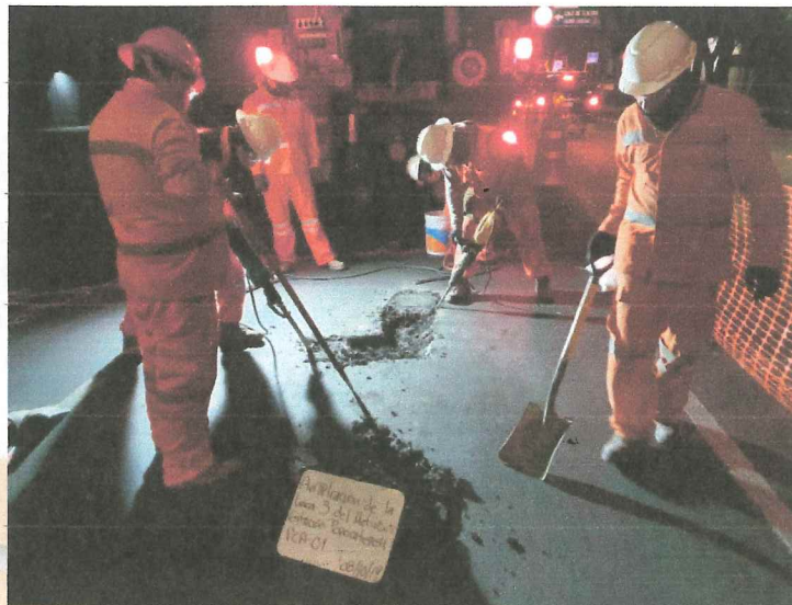
Figura 2.1. Vista de la excavación del PCA-01
