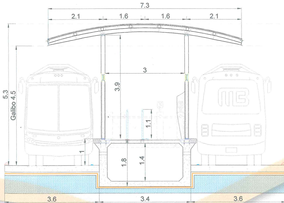
Figura 1.4. Vista en corte de la estación Popocatepetl, tomando como referencia la información de las estaciones Eugenia y Estación Terminal Xoco (CEMEX, 2019)
