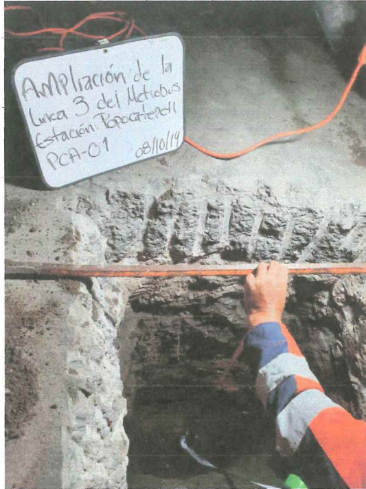
Figura 2.2. Muestreo y levantamiento geotécnico del PCA-01
