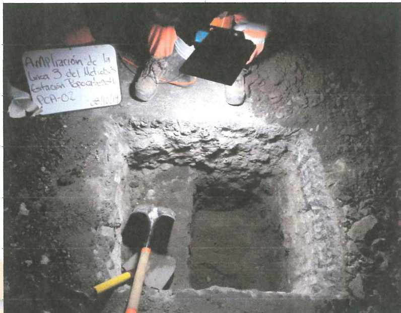
Figura 2.3. Vista de la excavación del PCA-02
