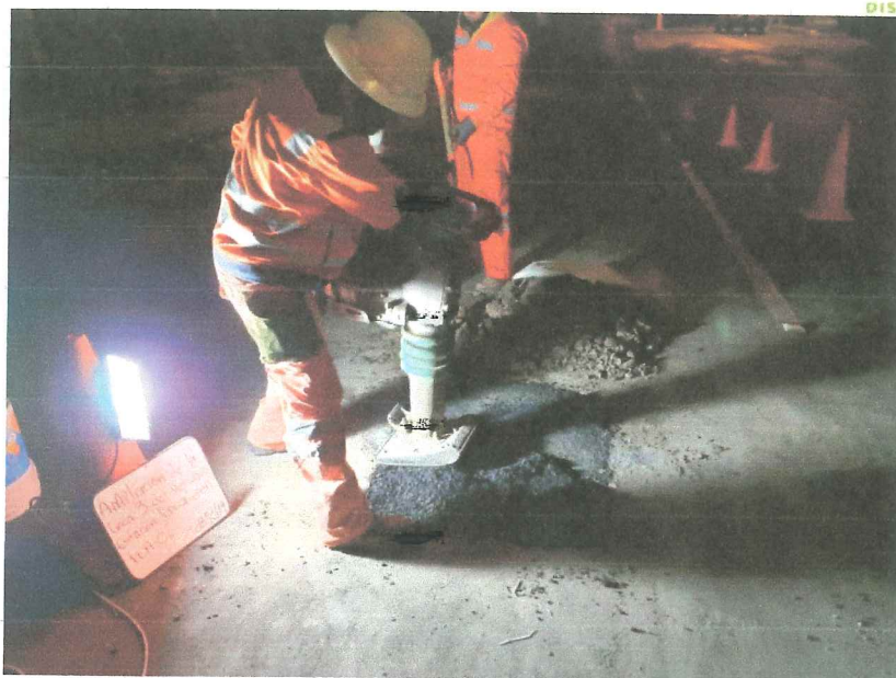
Figura 2.4. Relleno y compactación del PCA-02
