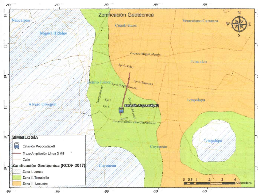
Figura 3.1. Zonificación geotécnica y localización de la estación Popocatepetl (RCDF, 2017)
