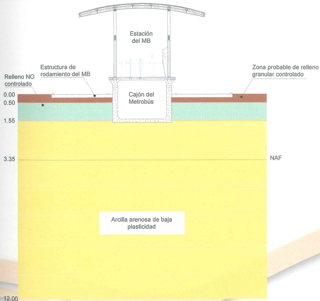
Figura 3.8 Modelo geotécnico propuesto para la estación del MB Popocatepetl
