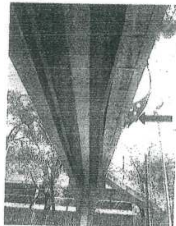
Imagen-9, Detalle trabe con reforzamiento externo.
