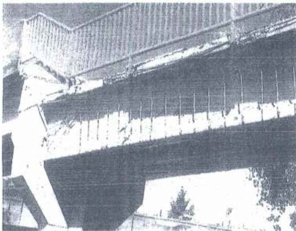
Imagen-7, Daño en alma y patín de la trabe, en lateral sur
