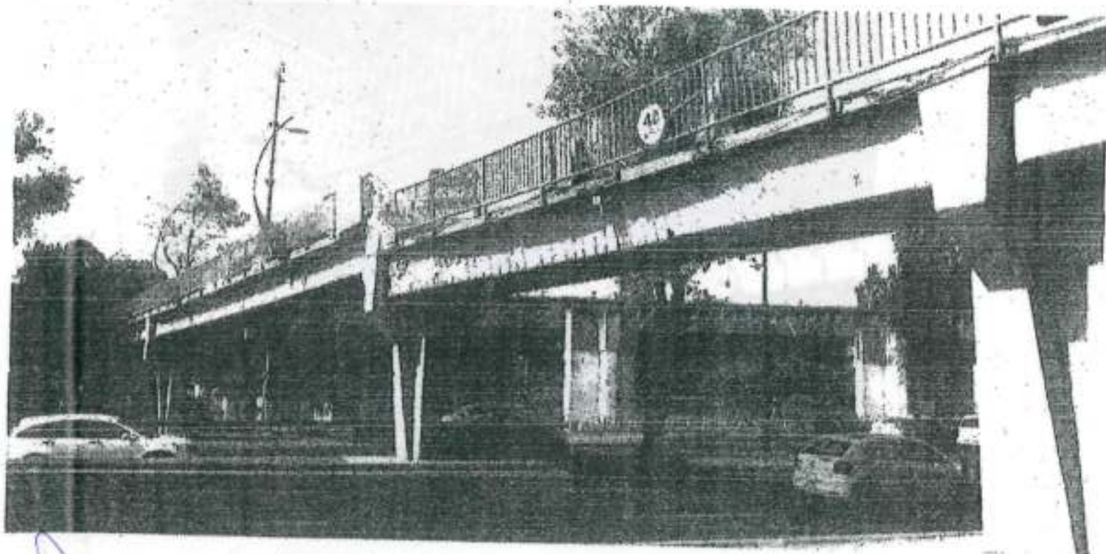
Imagen-6, Reforzamiento con estribos externos.
