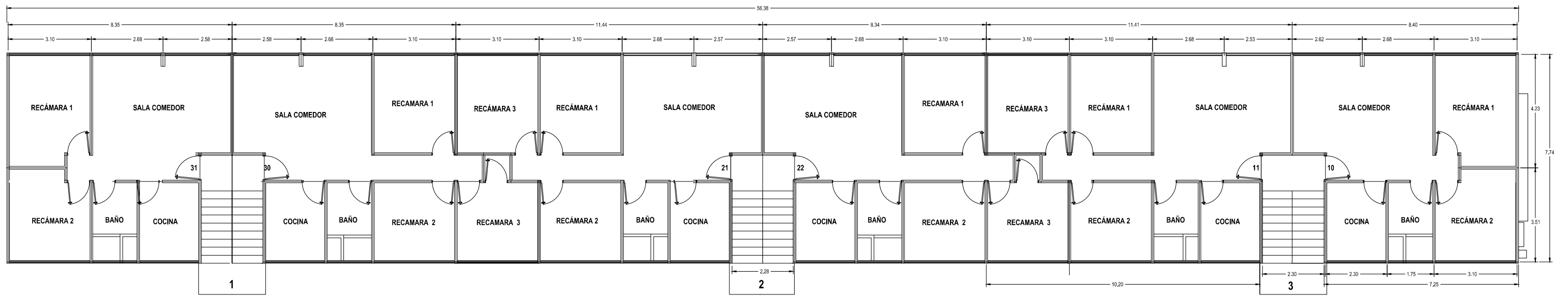
PLANTA BAJA MULTIFAMILIAR 4-A, 4-B y 4-C ESCALA:
